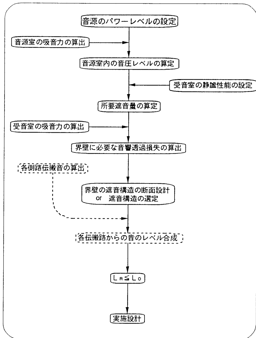
図-35 遮音設計手順の考え方の流れ
