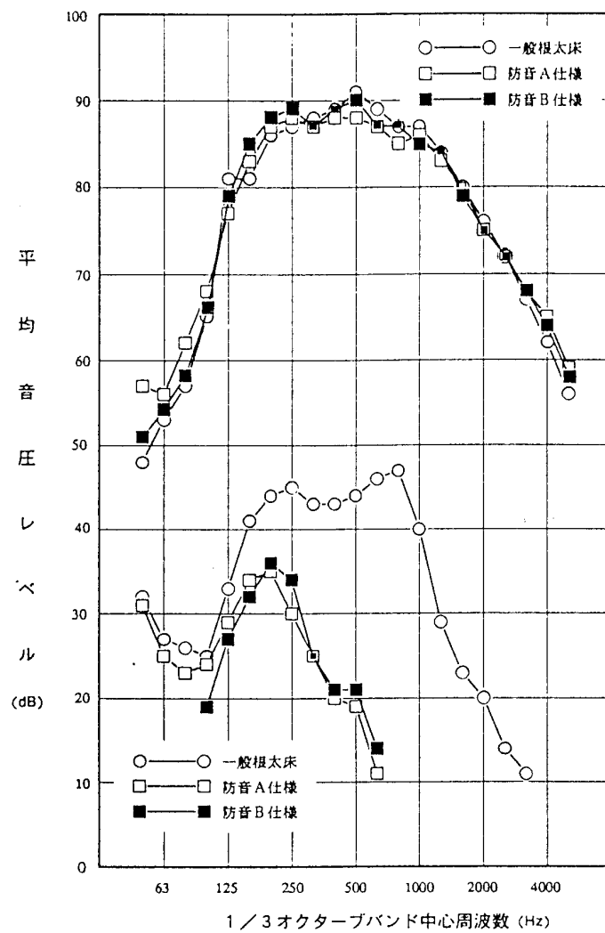
図-28 各防音仕様におけるピアノ演奏時室内発生音測定結果
